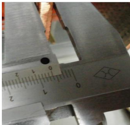
配电母排厚度照片
