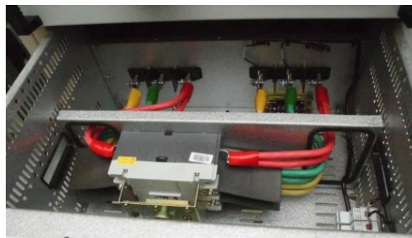
出线 7 抽屉照片
