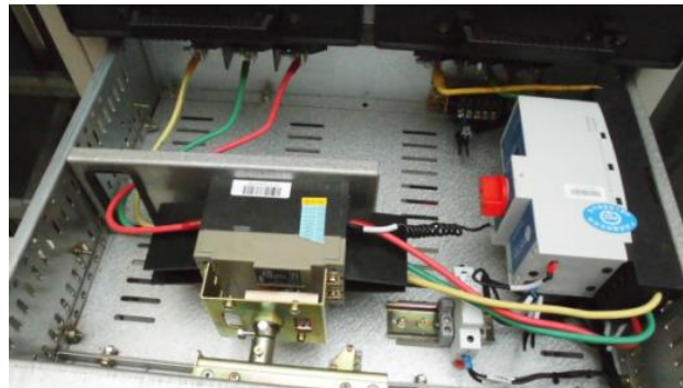
出线 5 抽屉照片
