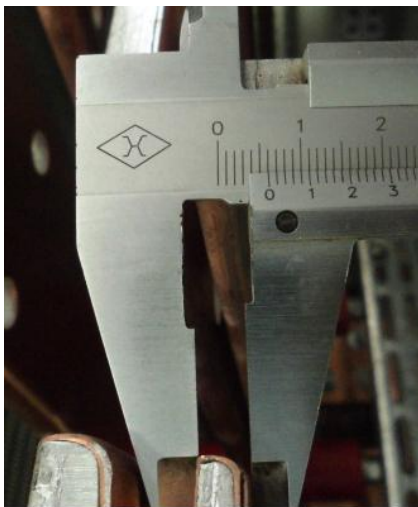
主开关进出线厚度（6mm）照片
