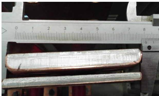
主开关进出线宽度照片
