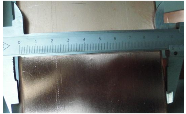
主母排宽度照片
