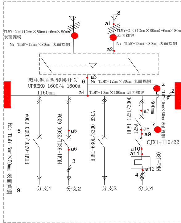
温升、短路点示意图 F1:
